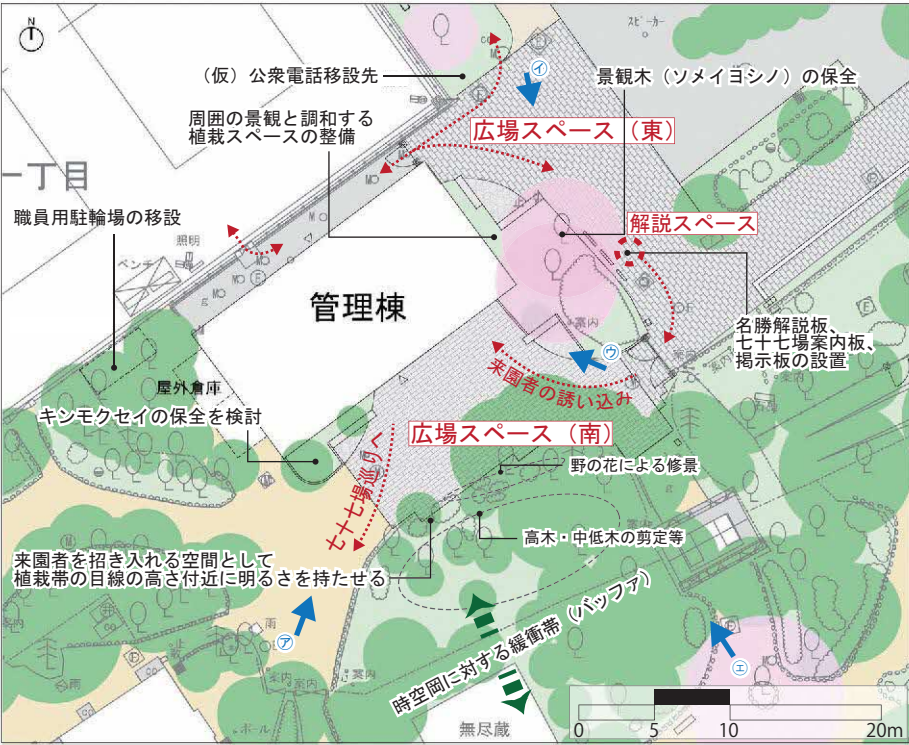
図3 外構計画の概要
