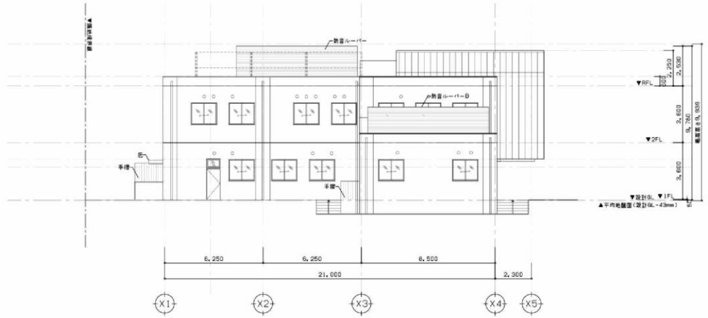
南立面图
