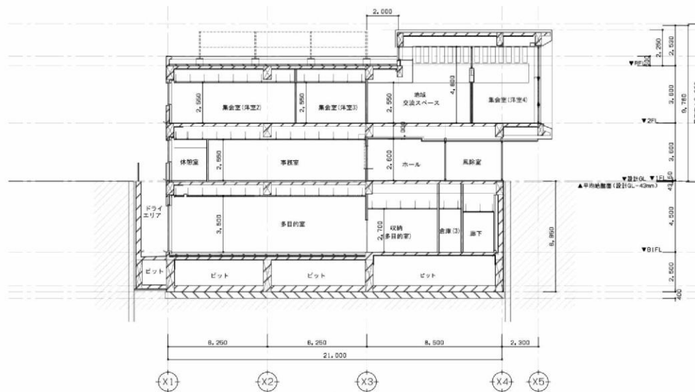
B-B'断面図
