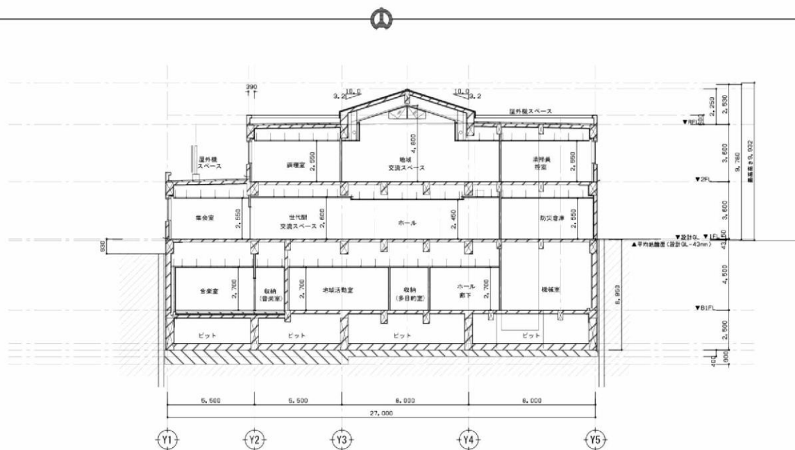
A-A'断面図
