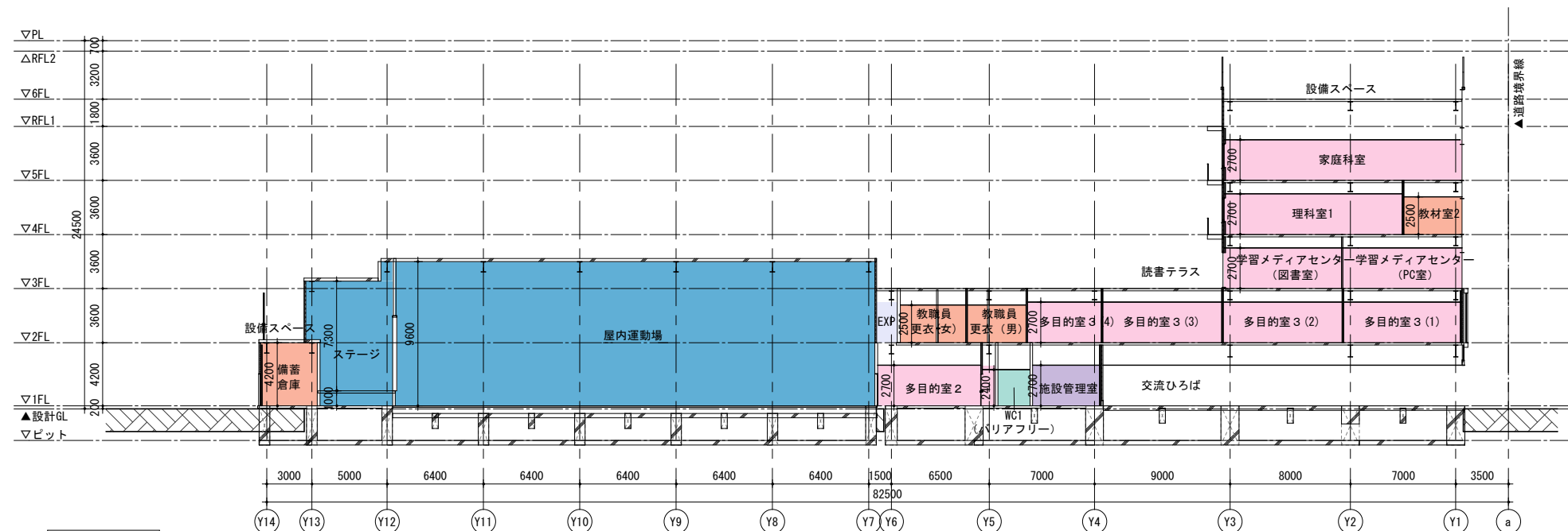
B-B' 断面図
