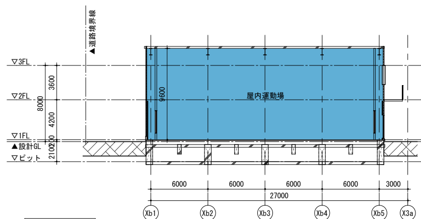
A-A' 断面図
